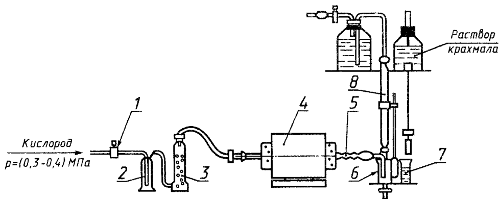
1 — кислородный баллон по ГОСТ 5583 с редукционным вентилем; 2 — склянка Тищенко, содержащая раствор марганцово-кислого калия массовой концентрации 0,04 г/см 3 в растворе гидроксида калия массовой концентрации 0,4 г/см 3 ; 3 — сушильная колонка, заполненная хлористым кальцием; 4 — трубчатая печь с карборундовыми нагревателями; 5 — фарфоровая (высокоглиноземистая) трубка длиной 750—800 мм и внутренним диаметром 20—26 мм; 6 — сосуд для титрования; 7 — сосуд для сравнения; 8 — бюретка
